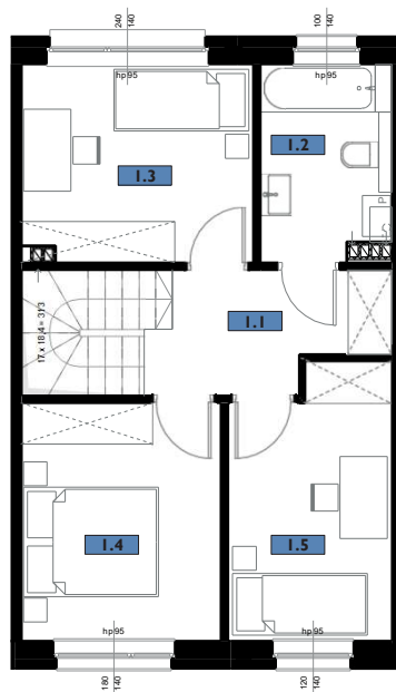
PIĘTRO
